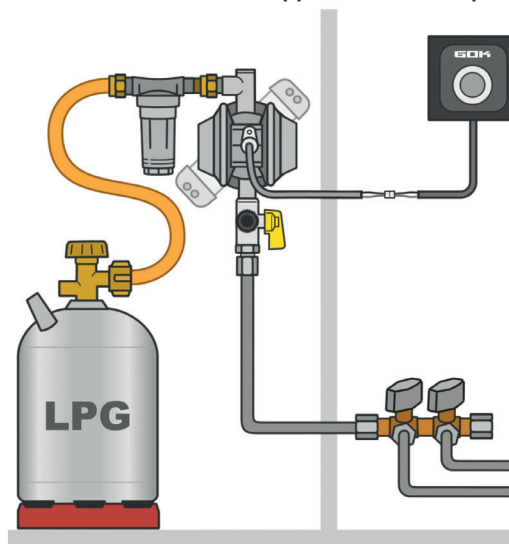
Caramatic BasicOne con apparecchiatura di prova
