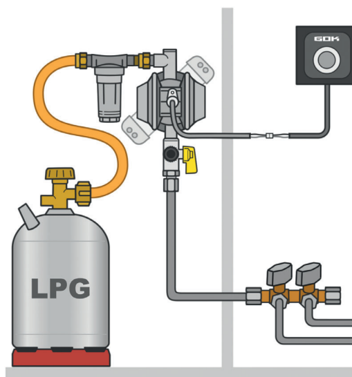
Caramatic BasicOne mit Prüfeinrichtung
