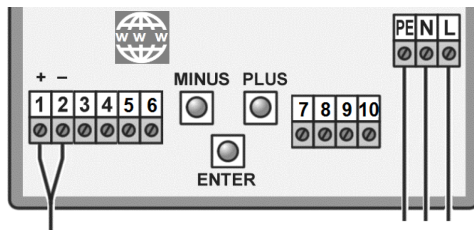
SmartBox 4 LAN
