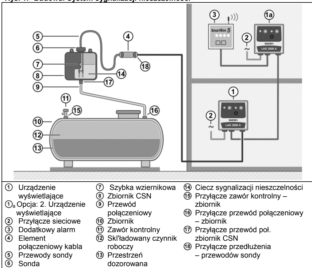
Rys. 1: Budowa: System sygnalizacji nieszczelności
